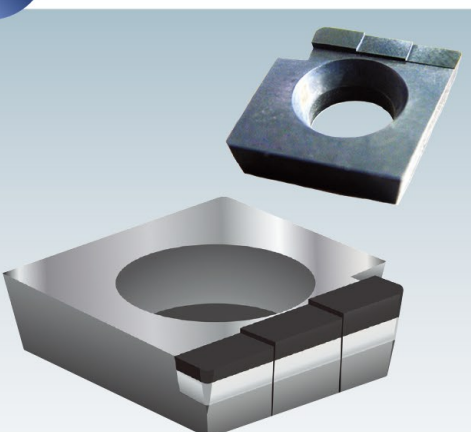
面加工時の切粉トラブルを解消する為に切刃を三段形状にした精密特殊ブレーカ。 切粉を縦に分断。
