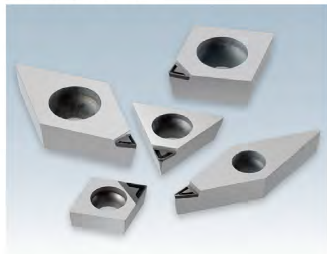
ブレーカ付PCDインサート
