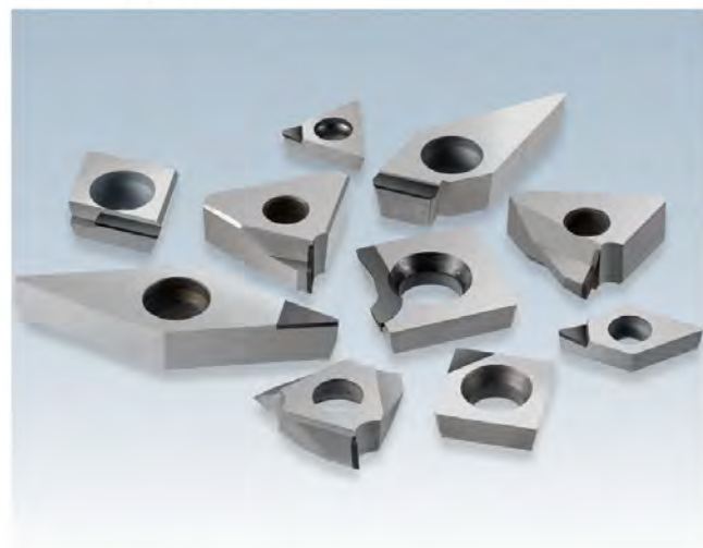
PCD/PcBN バイト PCD/PcBN ボーリングバイト PCD/PcBN カートリッジ
